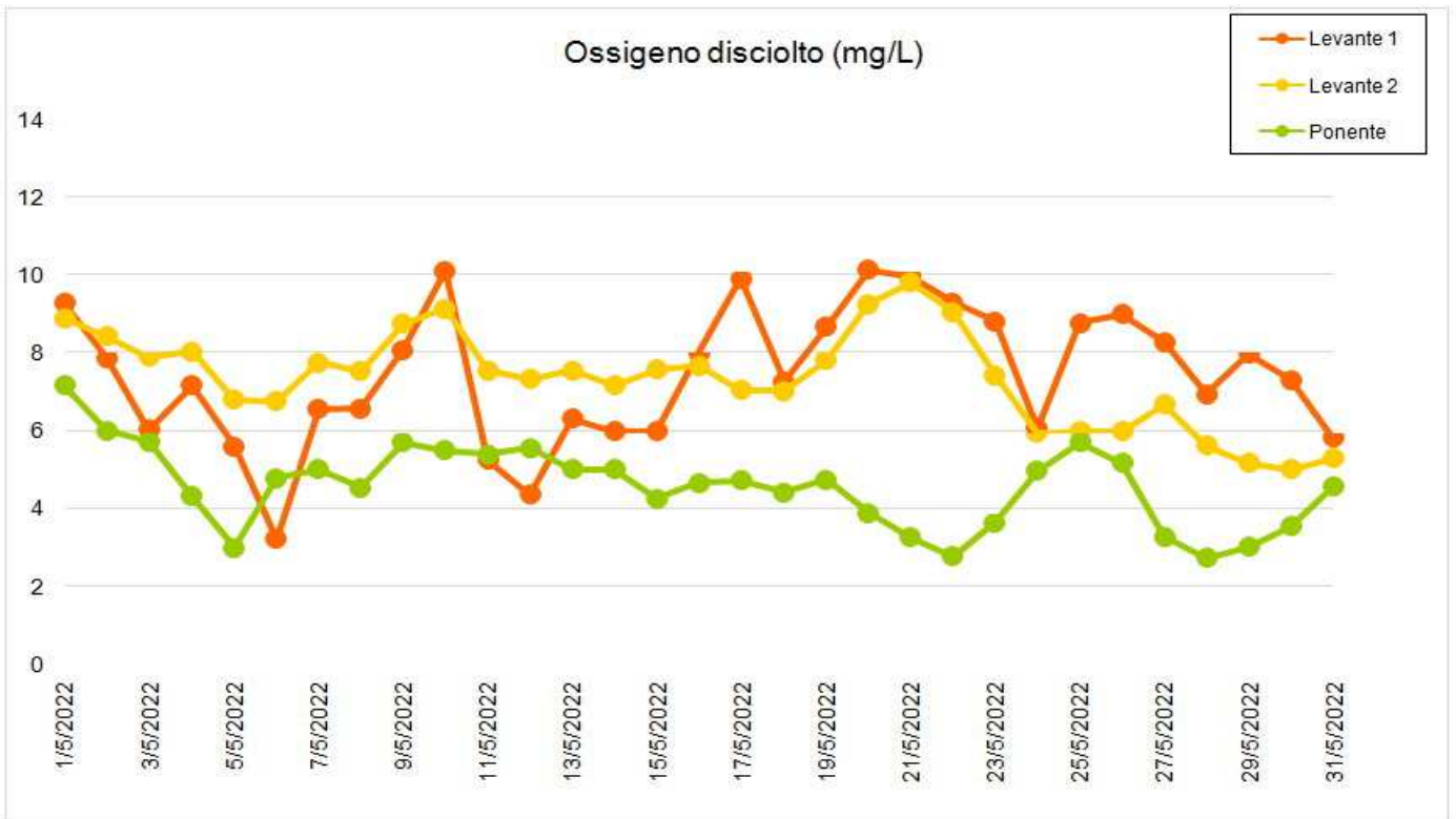
Figura 7 - Andamento dell'Ossigeno disciolto nella Laguna di Orbetello.
