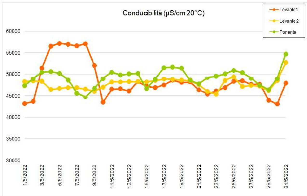
Figura 4 - Andamento della Conducibilità nella Laguna di Orbetello.
