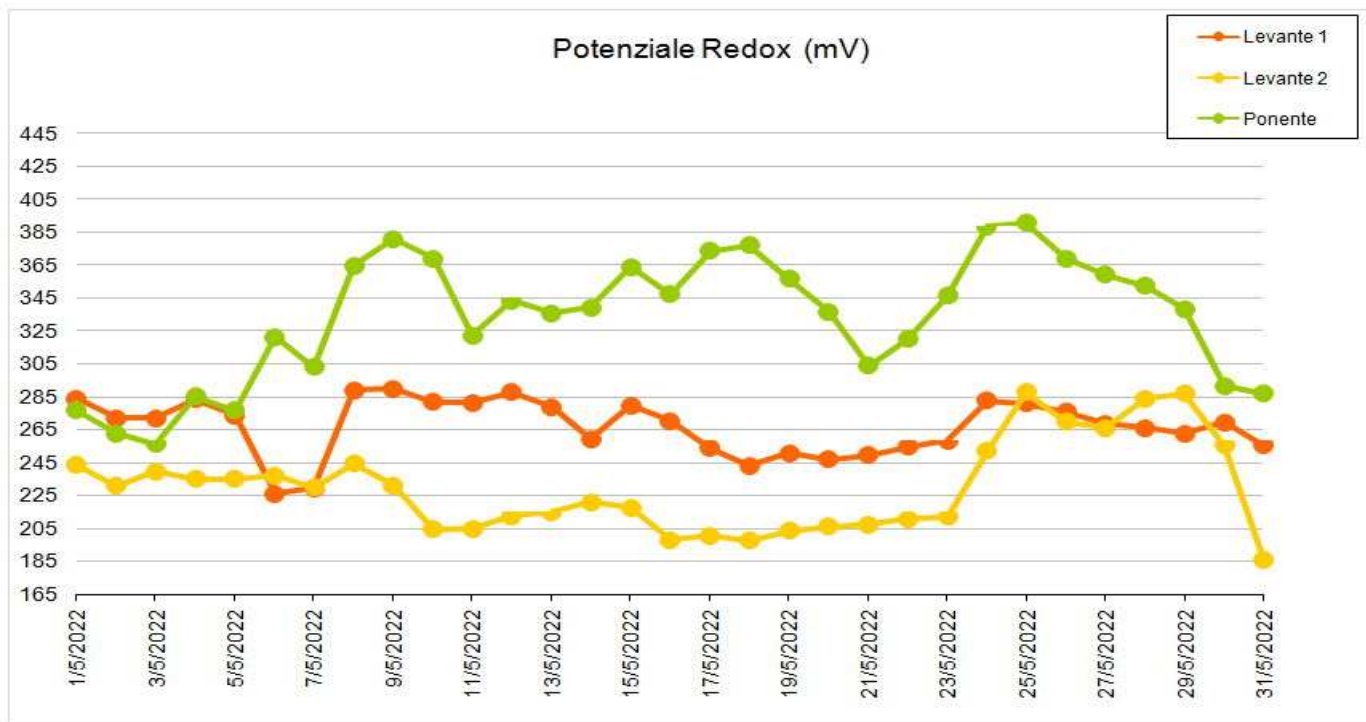
Figura 5 - Andamento del Potenziale Redox nella Laguna di Orbetello.
