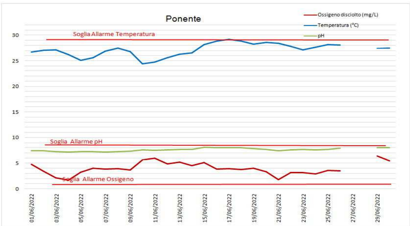
Figura 13 - Andamento e Soglie di Allarme per i parametri Temperatura, pH ed Ossigeno disciolto registrati dalla sonda multiparametrica Ponente.
