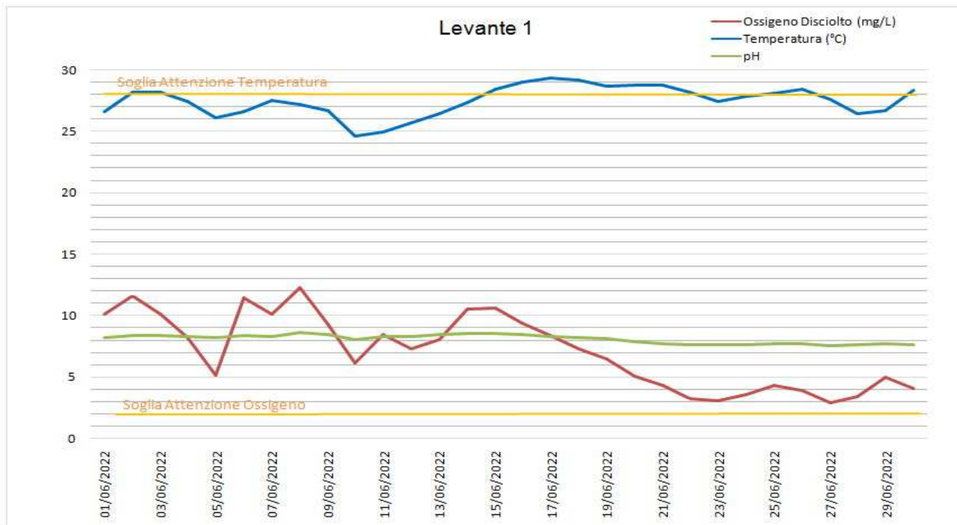
Figura 8 – Andamento e Soglie di Attenzione per i parametri Temperatura, pH, Ossigeno disciolto registrati dalla sonda multiparametrica Levante 1. Il pH non presenta Soglie di Attenzione (ma solo di Allarme).
