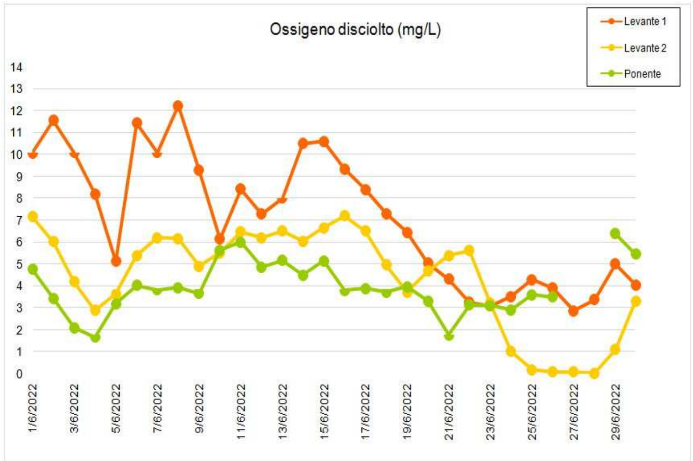
Figura 7 - Andamento dell'Ossigeno disciolto nella Laguna di Orbetello.
