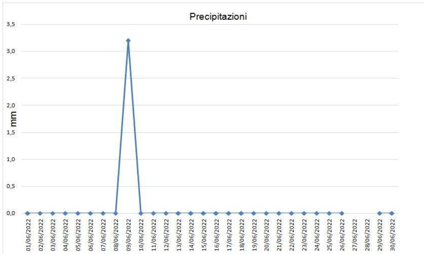
Figura 14 - Pluviometria della Laguna di Orbetello.
