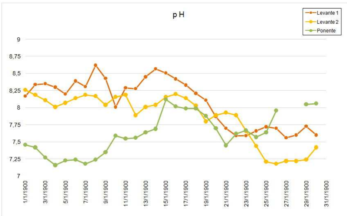
Figura 3 – Andamento del pH nella Laguna di Orbetello.
