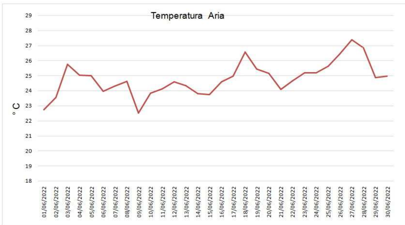
Figura 15 - Temperatura dell'aria sulla Laguna di Orbetello.
