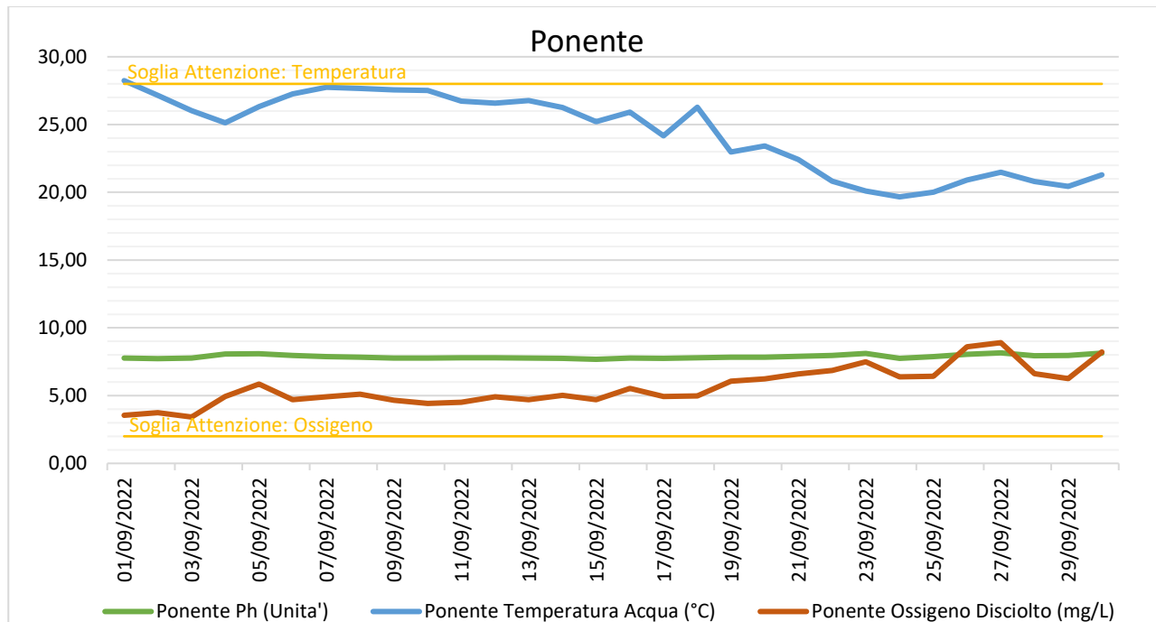
Figura 12 - Andamento medio giornaliero e Soglie di Attenzione per i parametri Temperatura, pH, Ossigeno disciolto registrati dalla sonda multiparametrica Ponente. Il pH non presenta Soglie di Attenzione (ma solo di Allarme).
