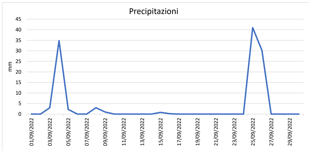
Figura 14 – Pluviometria media giornaliera della Laguna di Orbetello.
