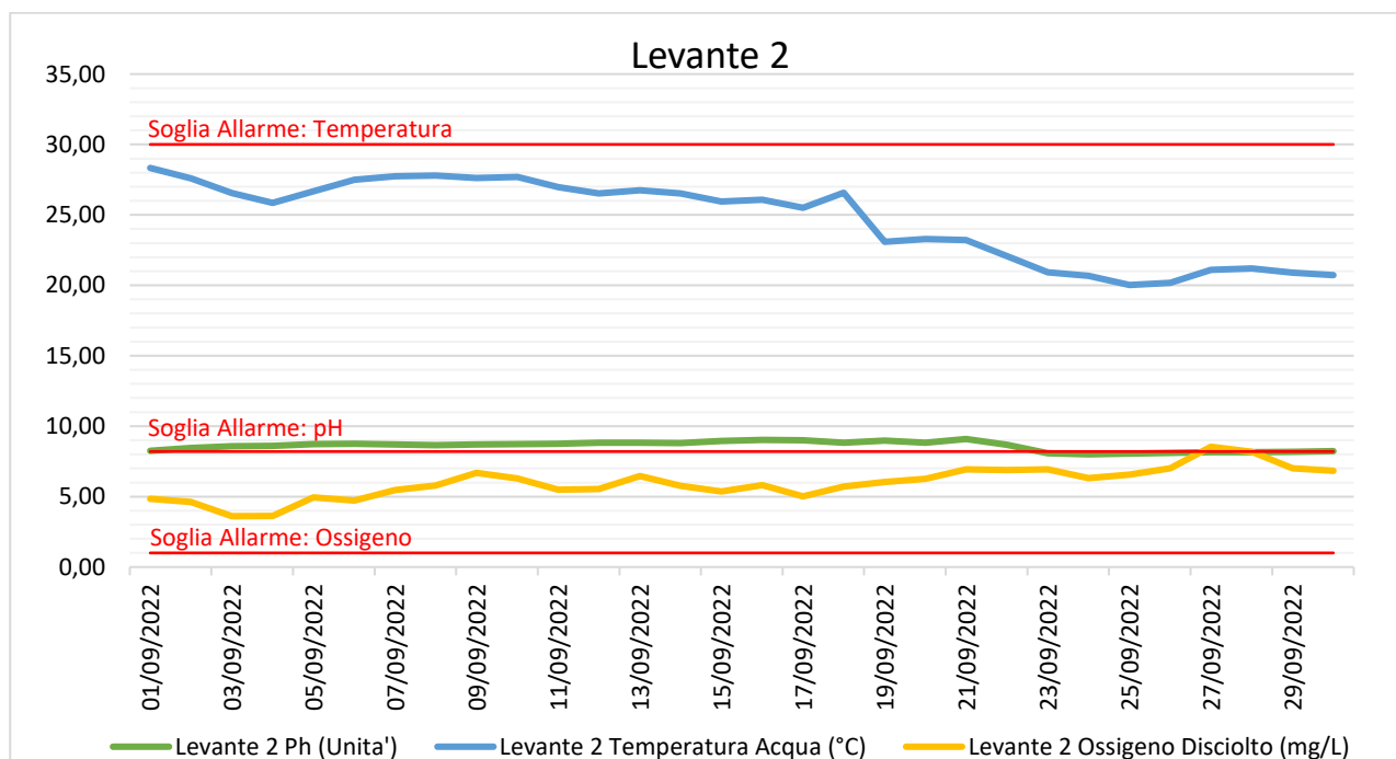
Figura 11 - Andamento medio giornaliero e Soglie di Allarme per i parametri Temperatura, pH ed Ossigeno disciolto registrati dalla sonda multiparametrica Levante 2.
