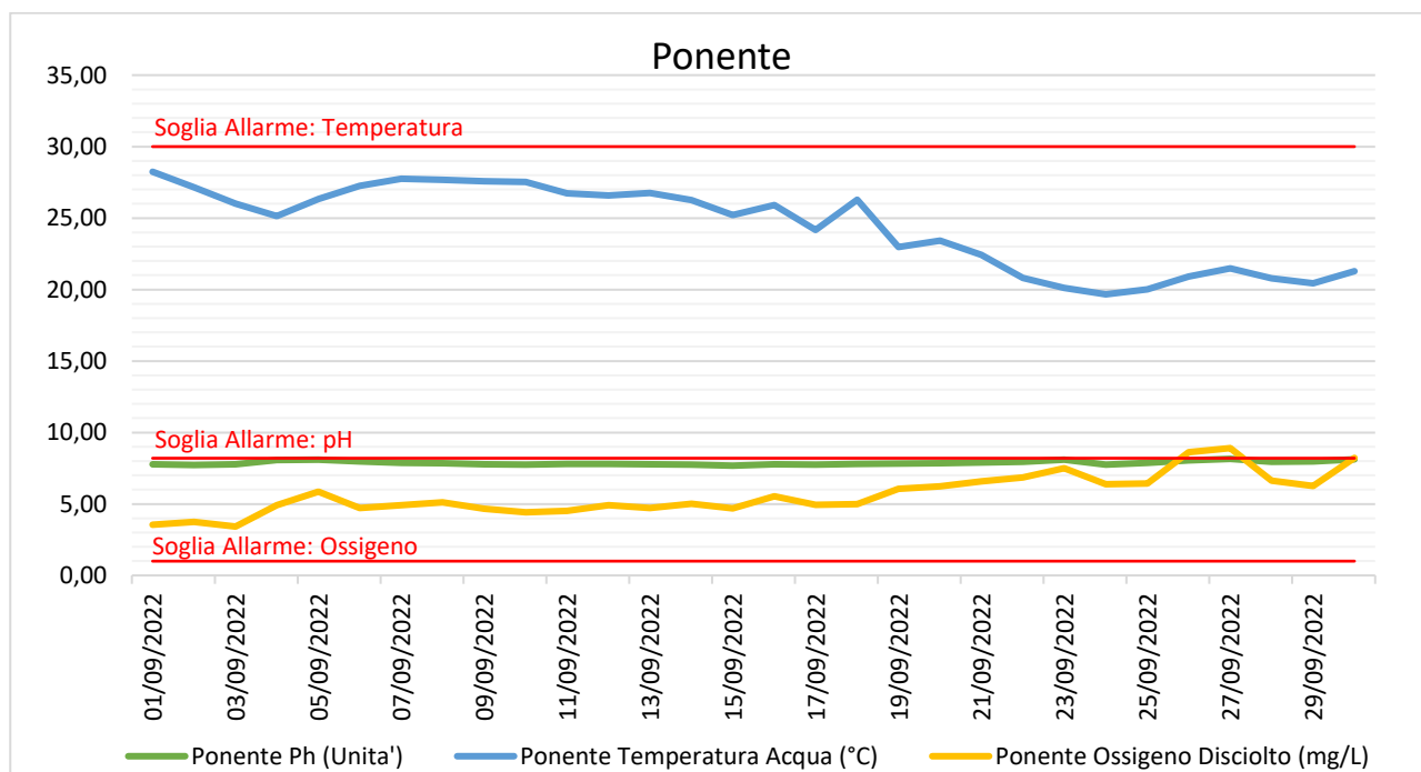
Figura 13 - Andamento medio giornaliero e Soglie di Allarme per i parametri Temperatura, pH ed Ossigeno disciolto registrati dalla sonda multiparametrica Ponente.
