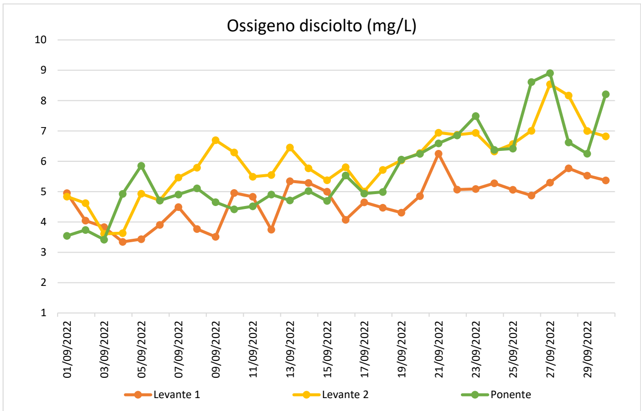
Figura 7 - Andamento medio giornaliero dell'Ossigeno disciolto nella Laguna di Orbetello.
