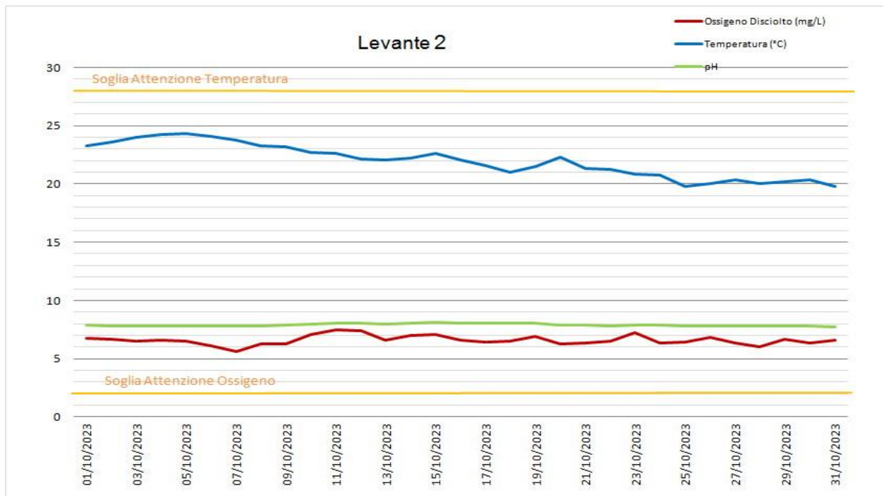
Figura 10 - Andamento medio giornaliero e Soglie di Attenzione per i parametri Temperatura, pH, Ossigeno disciolto registrati dalla sonda multiparametrica Levante 2. Il pH non presenta Soglie di Attenzione (ma solo di Allarme).
