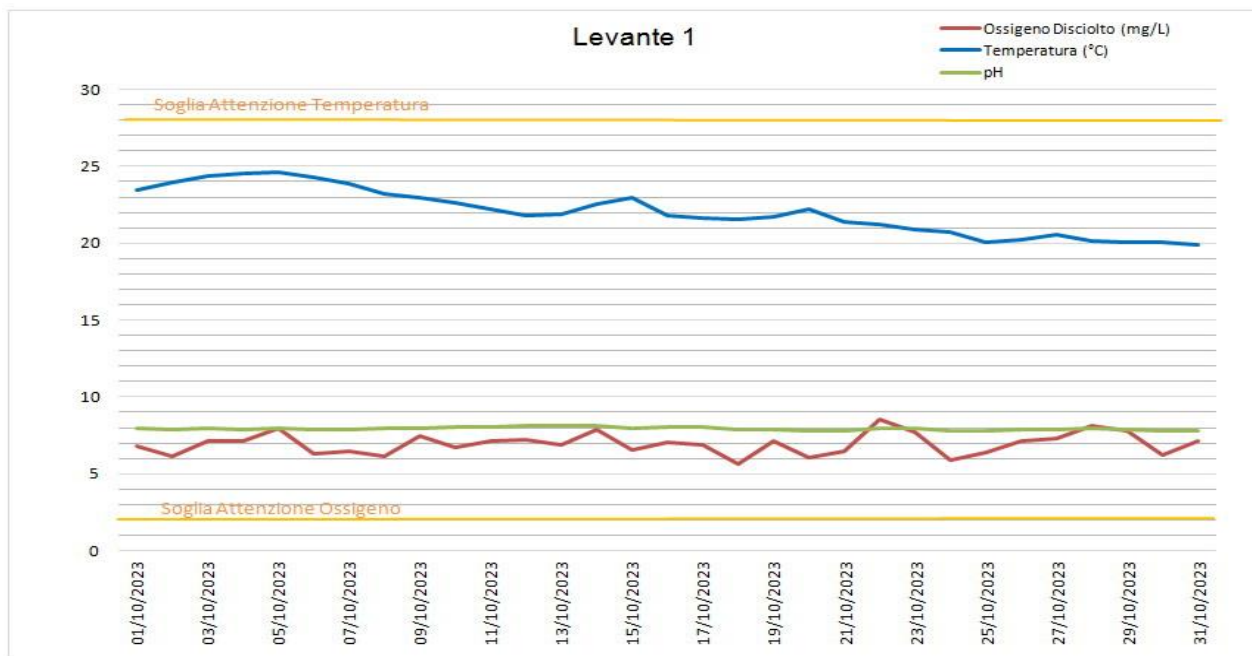
Figura 8 – Andamento medio giornaliero e Soglie di Attenzione per i parametri Temperatura, pH, Ossigeno disciolto registrati dalla sonda multiparametrica Levante 1. Il pH non presenta Soglie di Attenzione (ma solo di Allarme).
