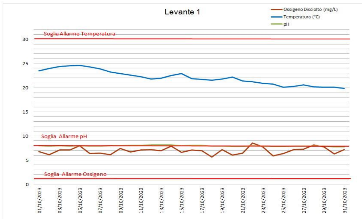
Figura 9 – Andamento medio giornaliero e Soglie di Allarme per i parametri Temperatura, pH ed Ossigeno disciolto registrati dalla sonda multiparametrica Levante 1.
