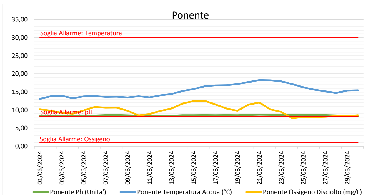
Figura 13 - Andamento medio giornaliero e Soglie di Allarme per i parametri Temperatura, pH ed Ossigeno disciolto registrati dalla sonda multiparametrica Ponente.
