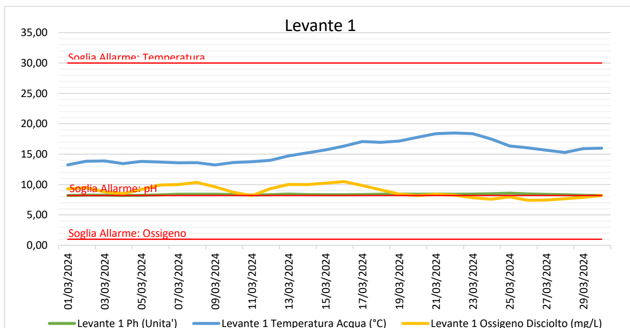
Figura 9 – Andamento medio giornaliero e Soglie di Allarme per i parametri Temperatura, pH ed Ossigeno disciolto registrati dalla sonda multiparametrica Levante 1.
