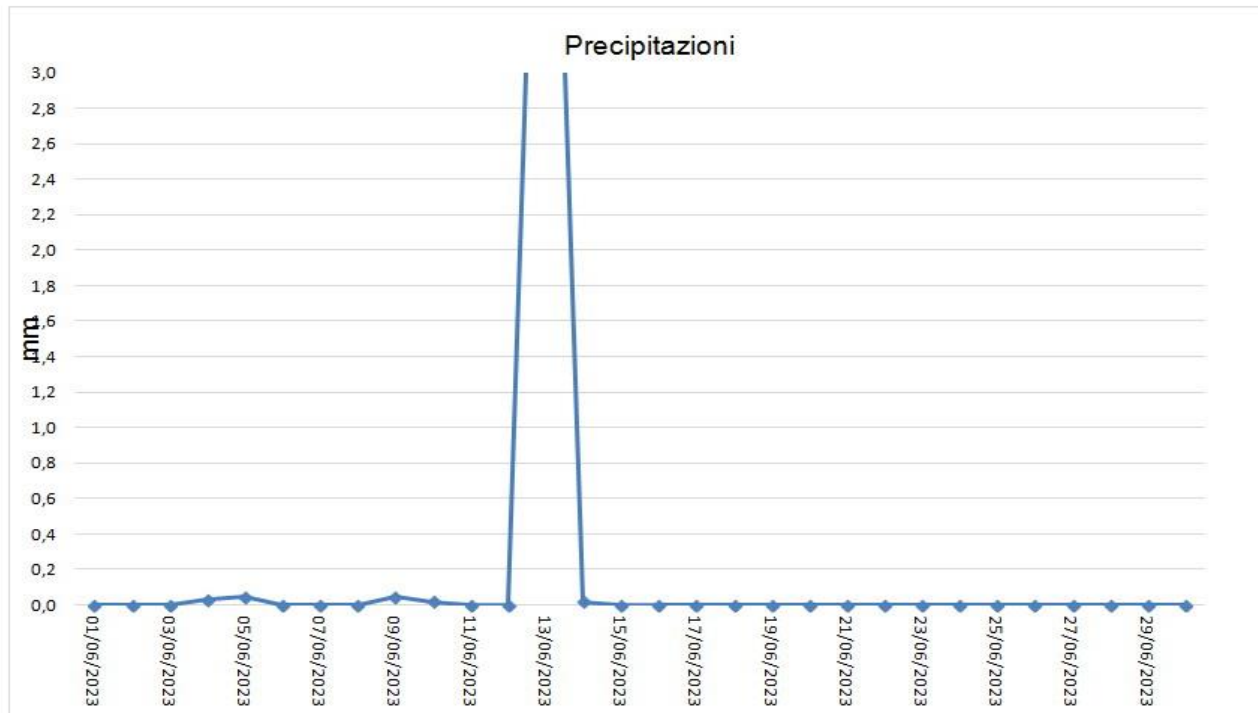
Figura 14 – Pluviometria media giornaliera della Laguna di Orbetello.
