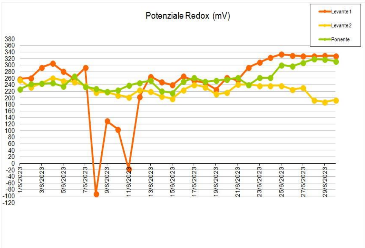
Figura 5 - Andamento medio giornaliero del Potenziale Redox nella Laguna di Orbetello.
