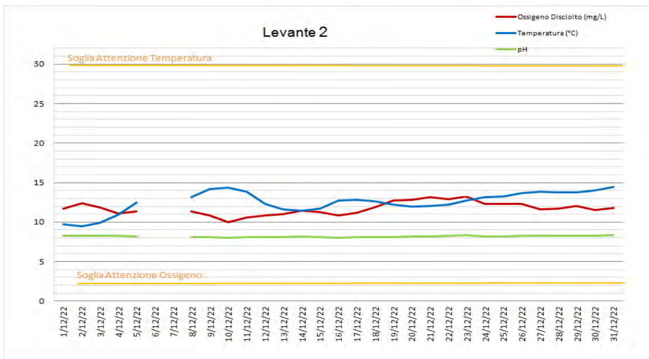
Figura 10 - Andamento e Soglie di Attenzione per i parametri Temperatura, pH, Ossigeno disciolto registrati dalla sonda
