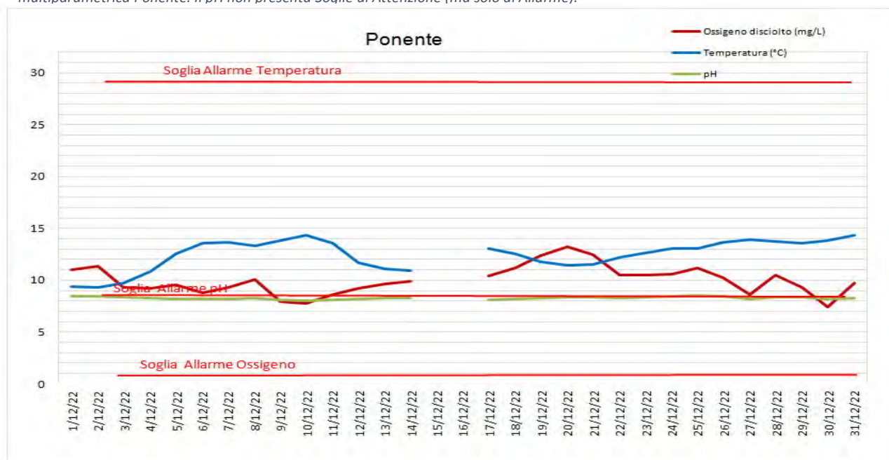
Figura 13 - Andamento e Soglie di Allarme per i parametri Temperatura, pH ed Ossigeno disciolto registrati dalla sonda multiparametrica Ponente.
