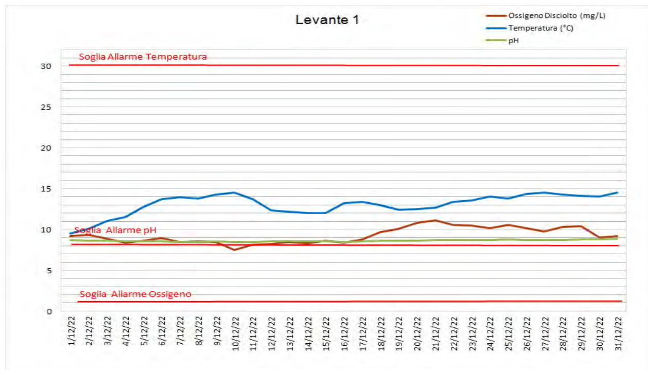
Figura 9 – Andamento e Soglie di Allarme per i parametri Temperatura, pH ed Ossigeno disciolto registrati dalla sonda multiparametrica Levante 1
