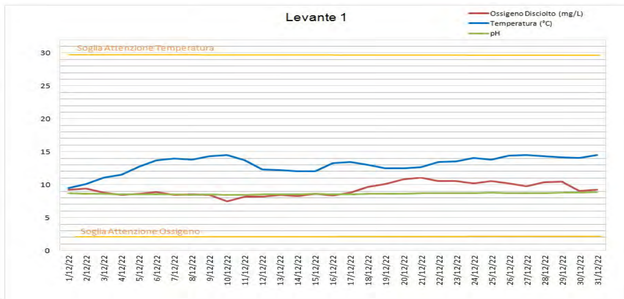
Figura 8 – Andamento e Soglie di Attenzione per i parametri Temperatura, pH, Ossigeno disciolto registrati dalla sonda multiparametrica Levante 1. Il pH non presenta Soglie di Attenzione (ma solo di Allarme).
