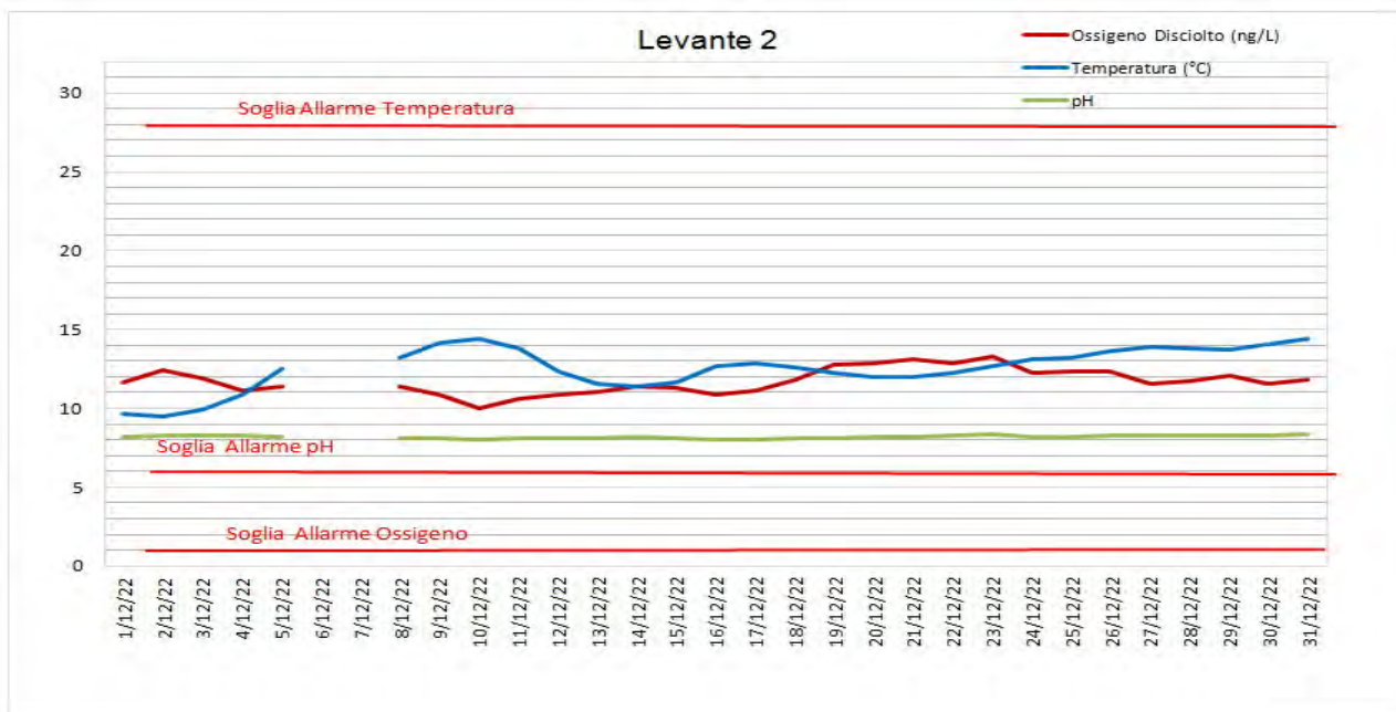
Figura 11 - Andamento e Soglie di Allarme per i parametri Temperatura, pH ed Ossigeno disciolto registrati dalla sonda multiparametrica Levante 2.
