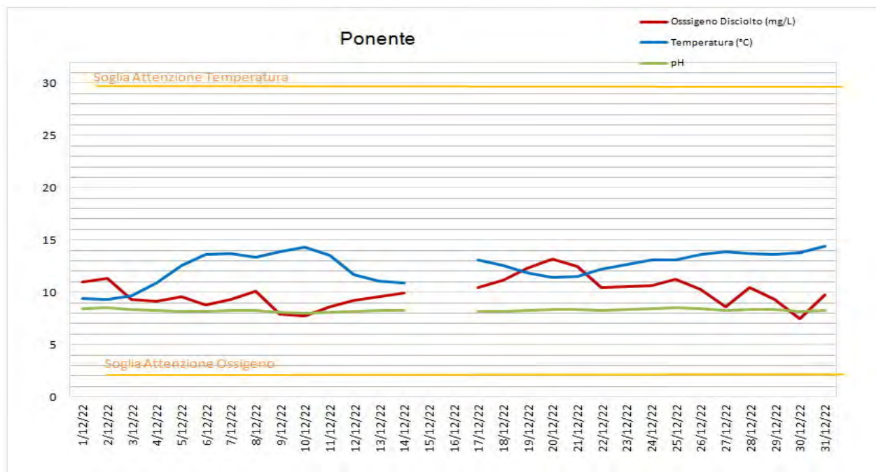
Figura 12 - Andamento e Soglie di Attenzione per i parametri Temperatura, pH, Ossigeno disciolto registrati dalla sonda multiparametrica Ponente. Il pH non presenta Soglie di Attenzione (ma solo di Allarme).
