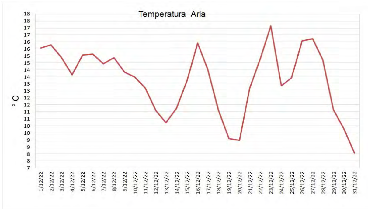
Figura 15 - Temperatura dell'aria sulla Laguna di Orbetello.
