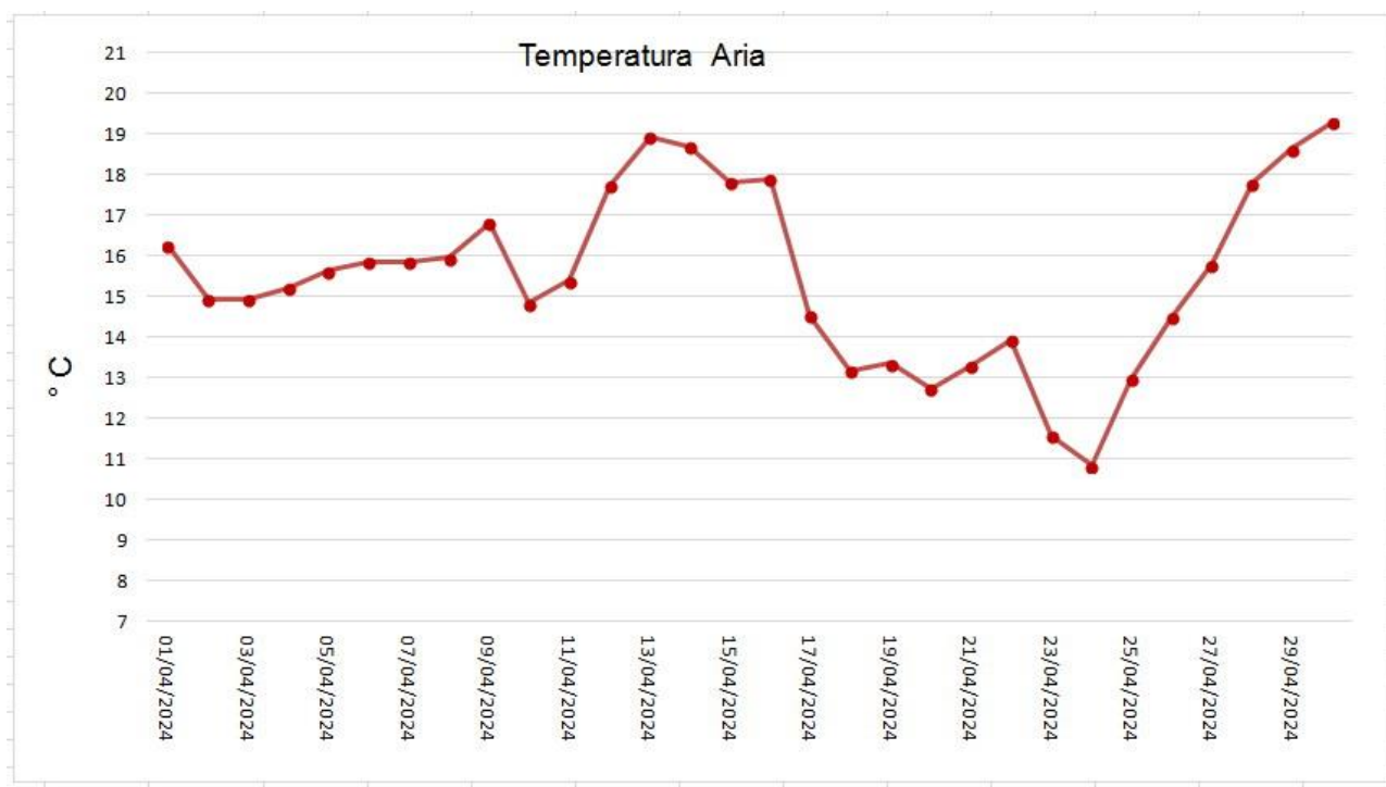
Figura 15 – Temperatura media giornaliera dell'aria sulla Laguna di Orbetello.
