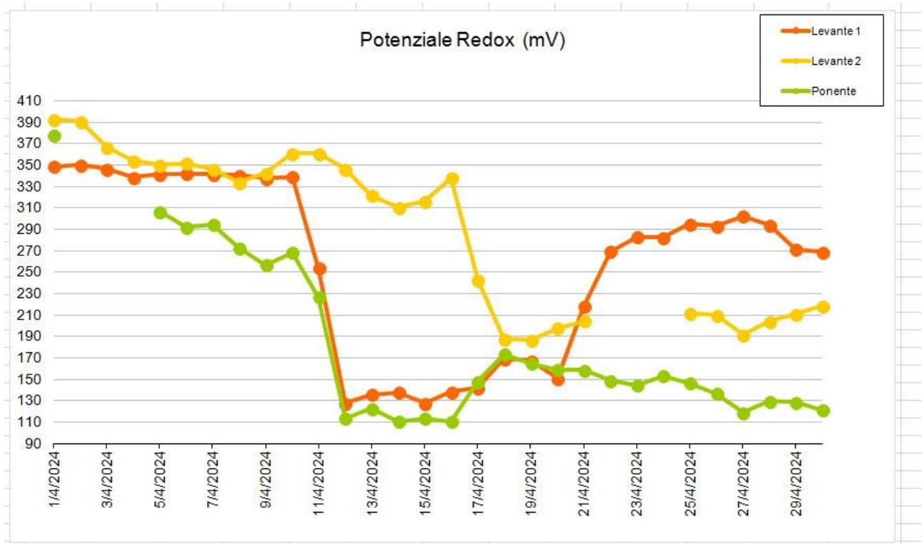
Figura 5 - Andamento medio giornaliero del Potenziale Redox nella Laguna di Orbetello.
