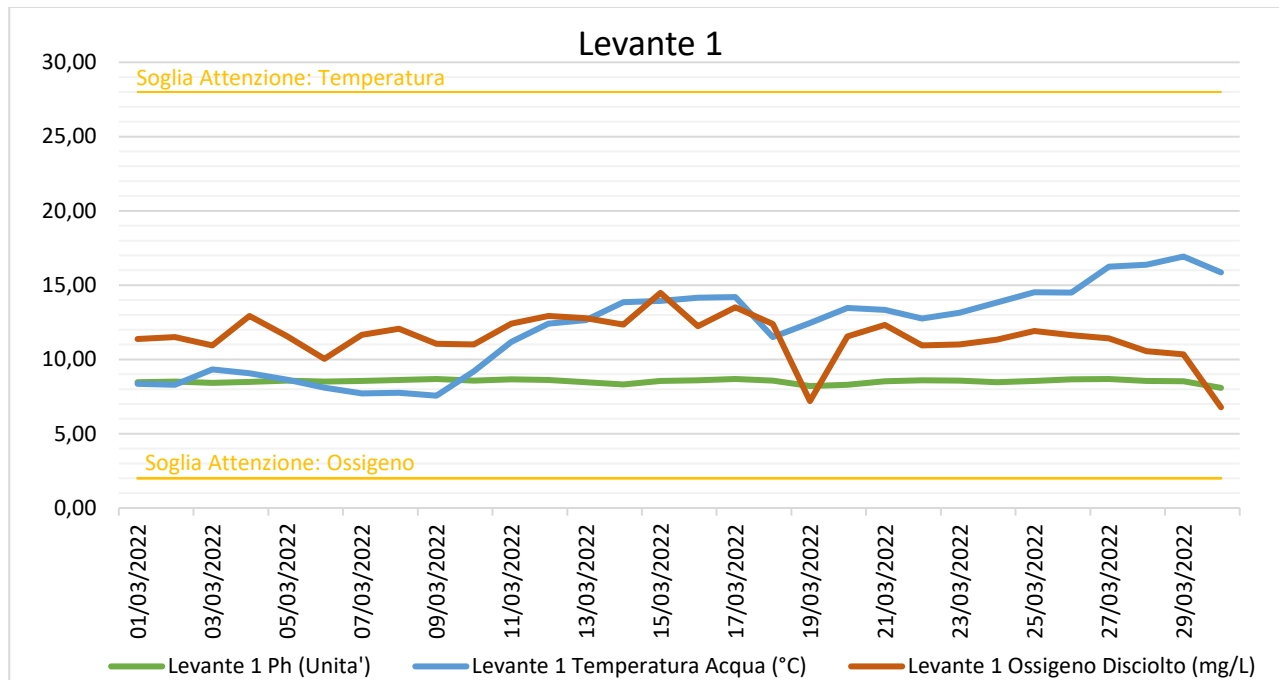
Figura 8 – Andamento e Soglie di Attenzione per i parametri Temperatura, pH, Ossigeno disciolto registrati dalla sonda multiparametrica Levante 1. Il pH non presenta Soglie di Attenzione (ma solo di Allarme).
