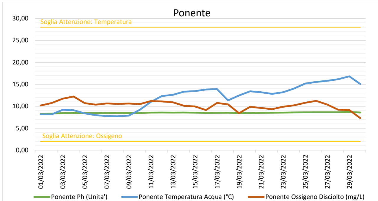
Figura 12 - Andamento e Soglie di Attenzione per i parametri Temperatura, pH, Ossigeno disciolto registrati dalla sonda multiparametrica Ponente. Il pH non presenta Soglie di Attenzione (ma solo di Allarme).
