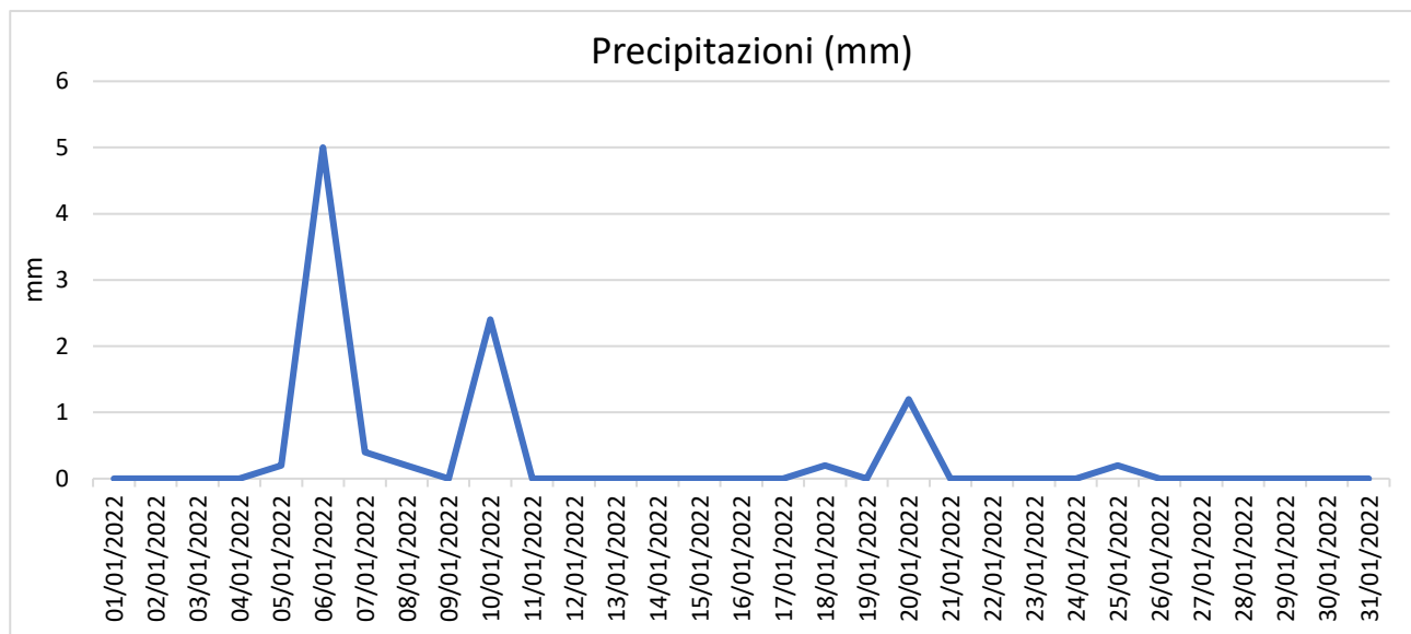
Figura 14 - Pluviometria della Laguna di Orbetello.
