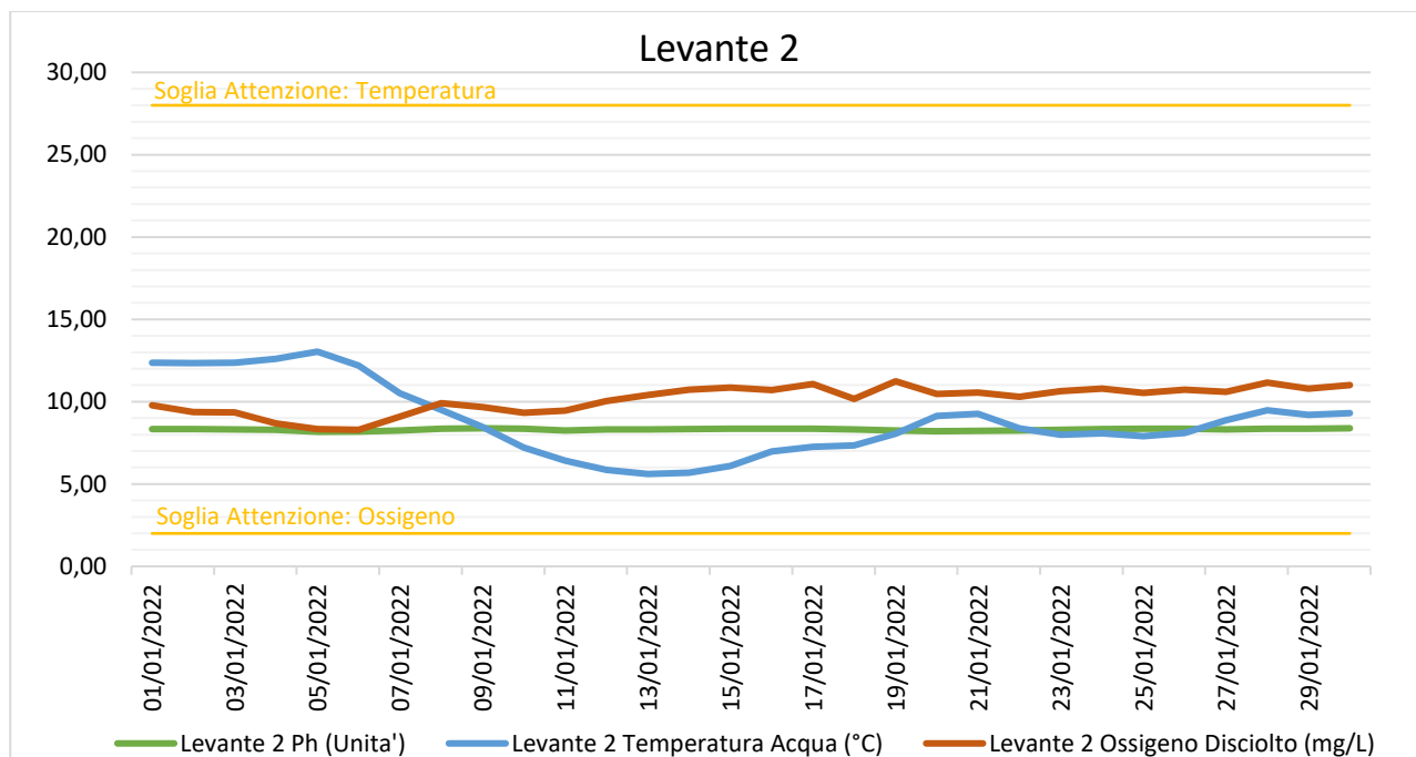
Figura 10 - Andamento e Soglie di Attenzione per i parametri Temperatura, pH, Ossigeno disciolto registrati dalla sonda multiparametrica Levante 2. Il pH non presenta Soglie di Attenzione (ma solo di Allarme).
