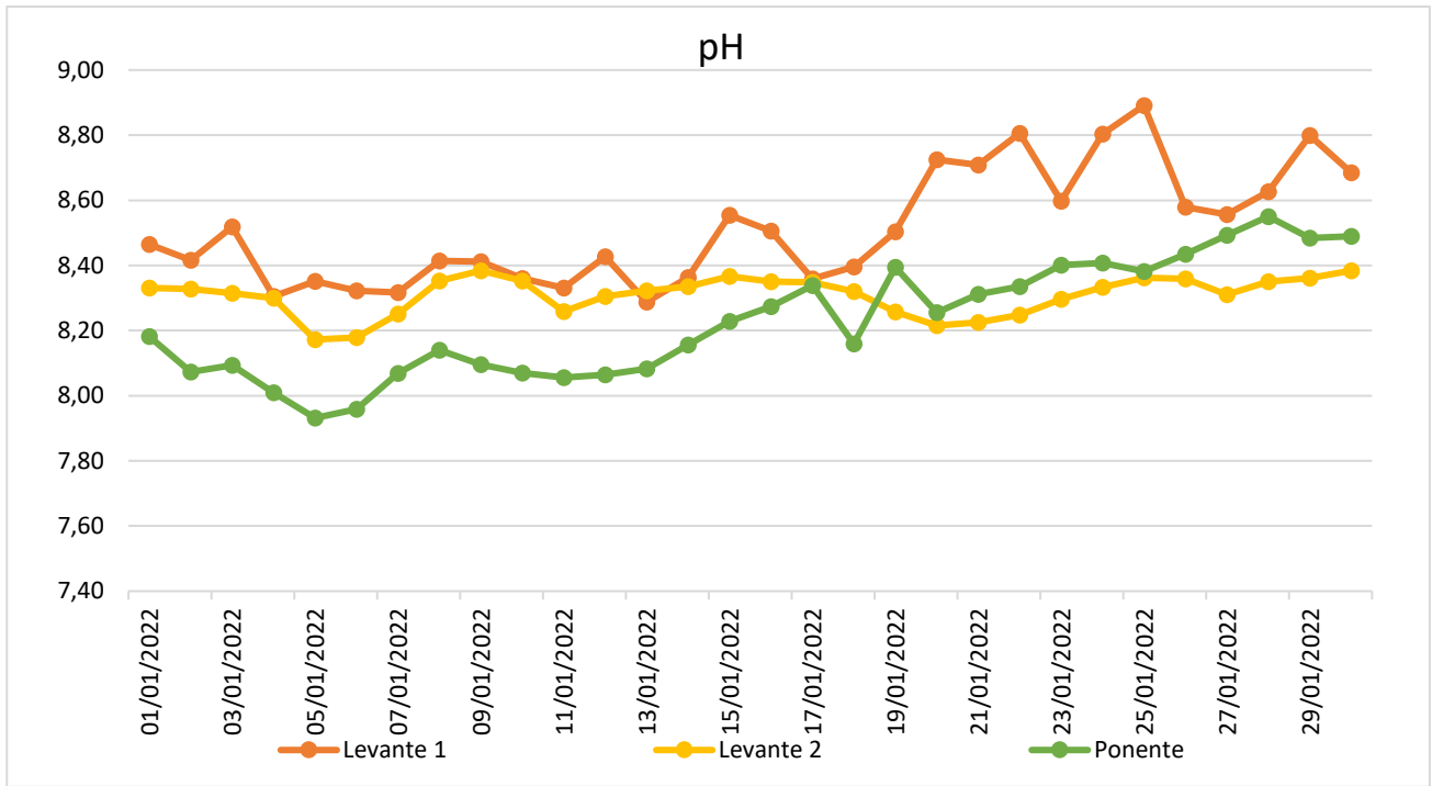
Figura 3 – Andamento del pH nella Laguna di Orbetello.
