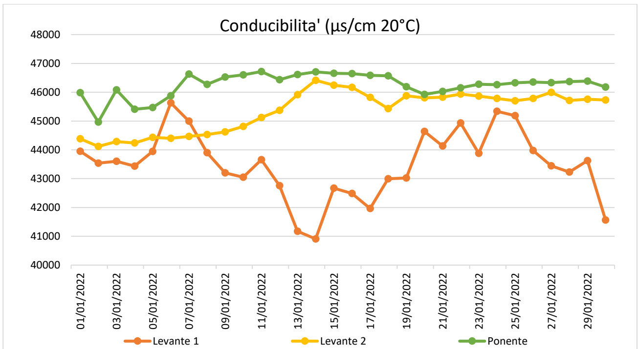
Figura 4 - Andamento della Conducibilità nella Laguna di Orbetello.
