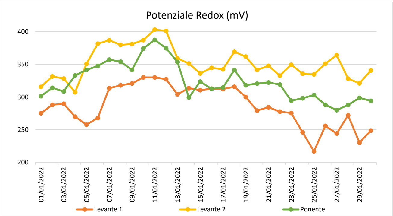
Figura 5 - Andamento del Potenziale Redox nella Laguna di Orbetello.
