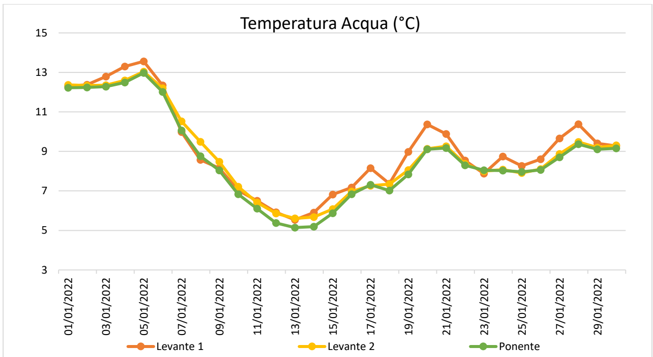
Figura 6 - Andamento della Temperatura dell'acqua nella Laguna di Orbetello.
