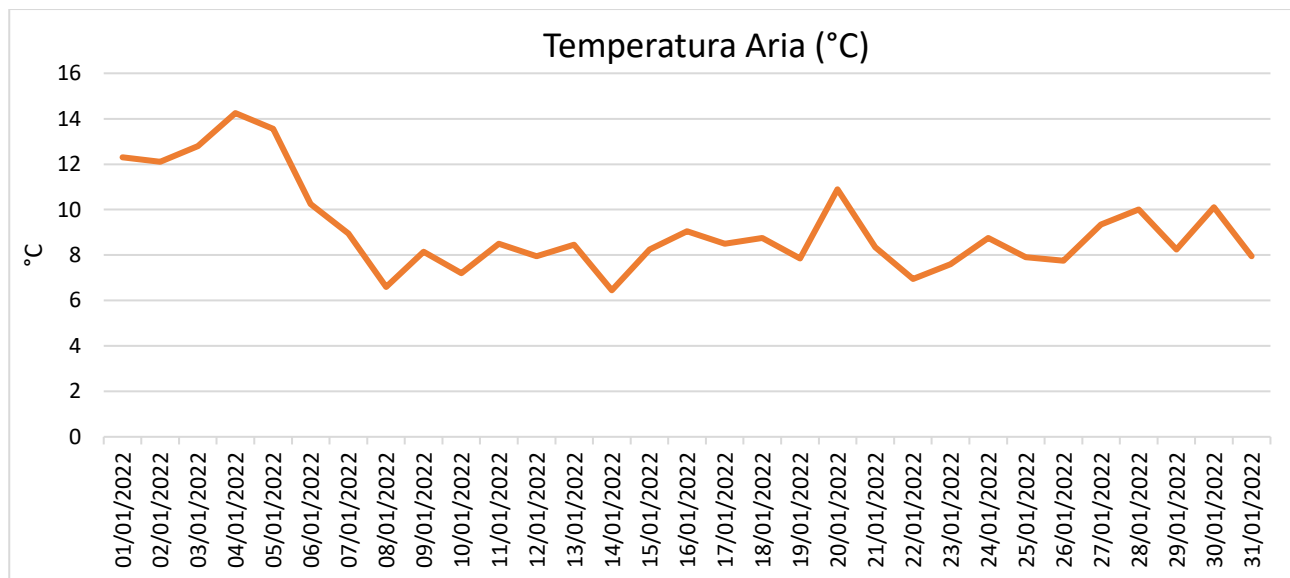
Figura 15 - Temperatura dell'aria sulla Laguna di Orbetello.
