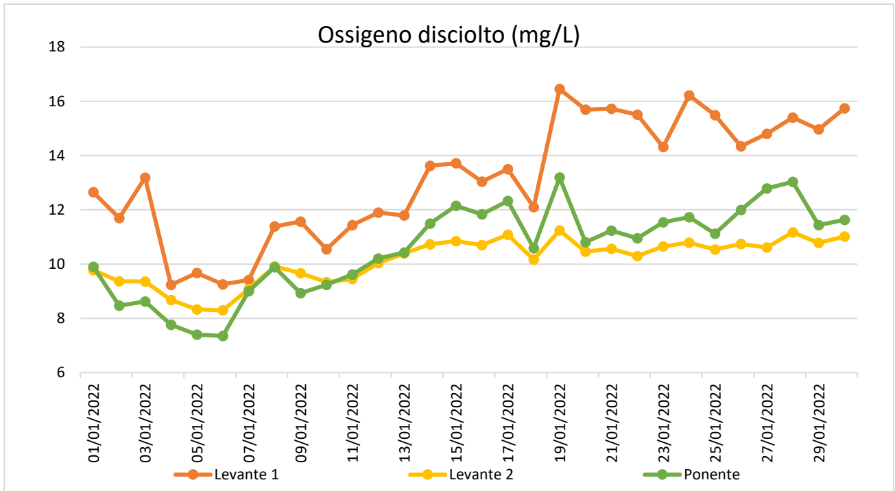
Figura 7 - Andamento dell'Ossigeno disciolto nella Laguna di Orbetello.
