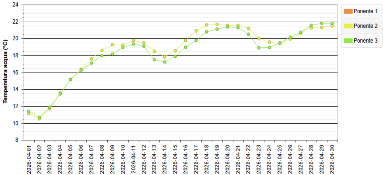
Figura 14 - Andamento medio giornaliero della Temperatura nella Laguna di Ponente.
