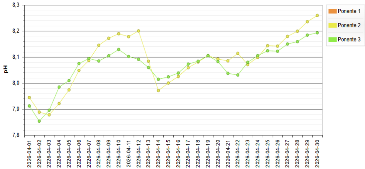
Figura 8 – Andamento medio giornaliero del pH nella Laguna di Ponente.
