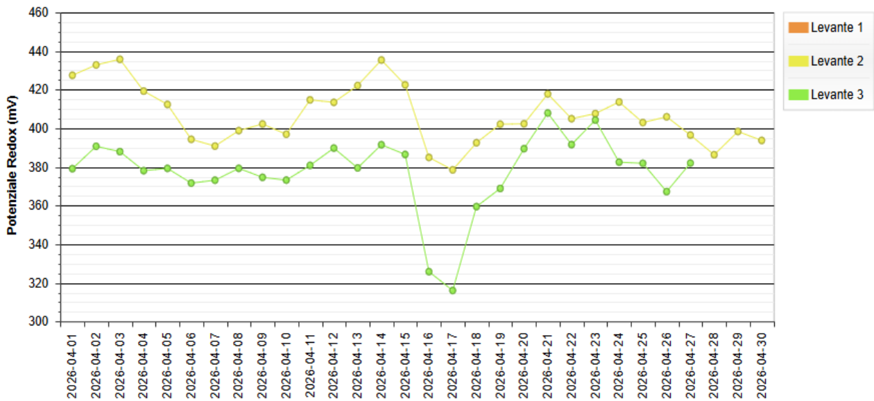
Figura 13 - Andamento medio giornaliero del Potenziale Redox nella Laguna di Levante.
