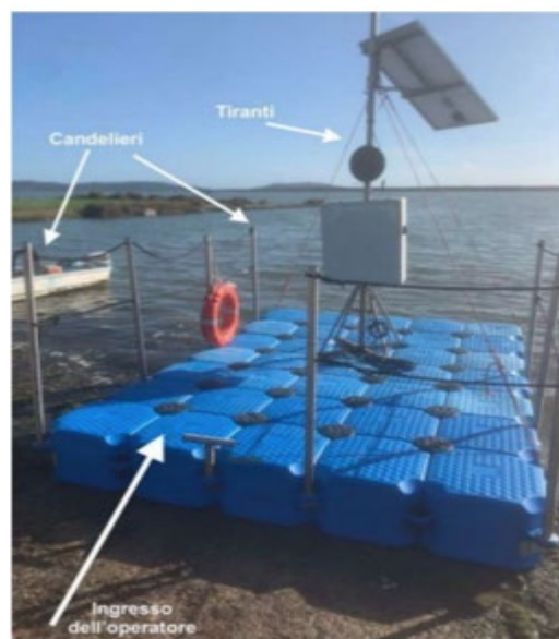
Figura 6 – Esempio di stazione di monitoraggio galleggiante posizionata nella Laguna di Orbetello
