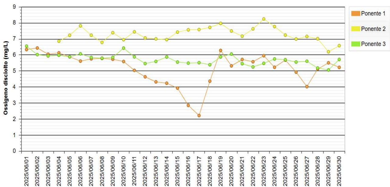
Figura 16 - Andamento medio giornaliero dell'Ossigeno disciolto nella Laguna di Ponente.
