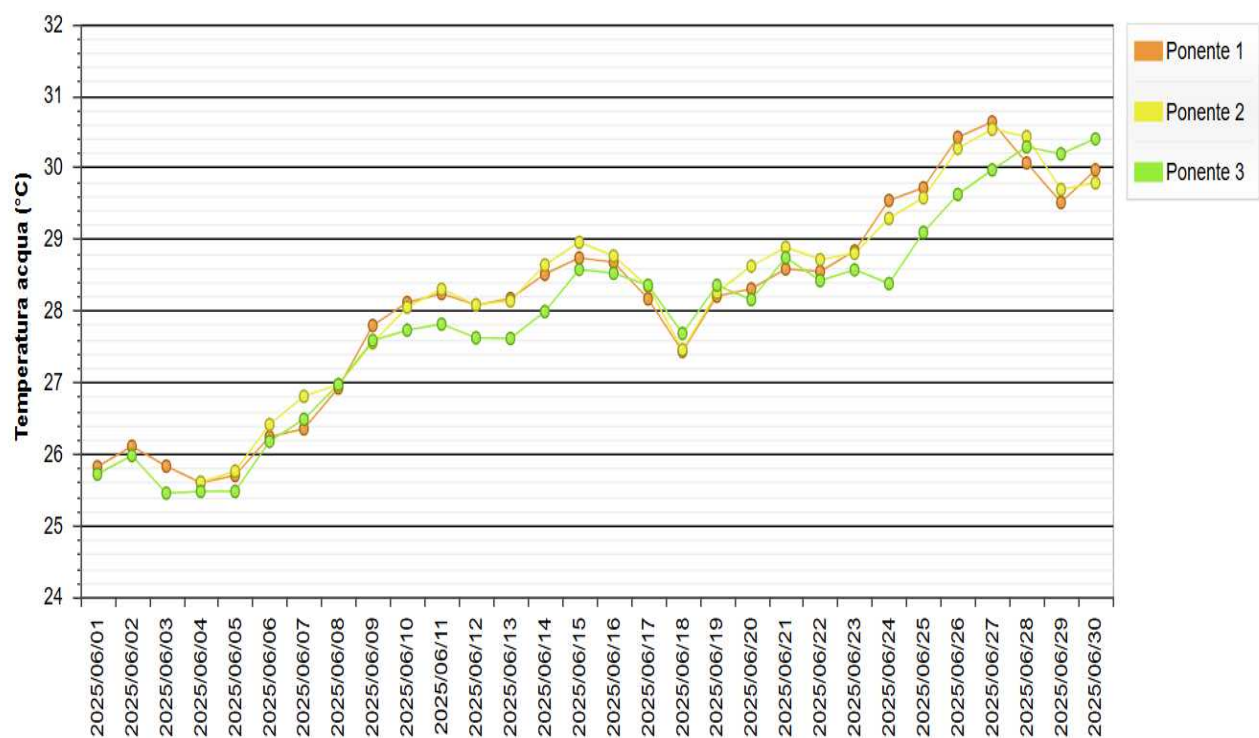
Figura 14 - Andamento medio giornaliero della Temperatura nella Laguna di Ponente.
