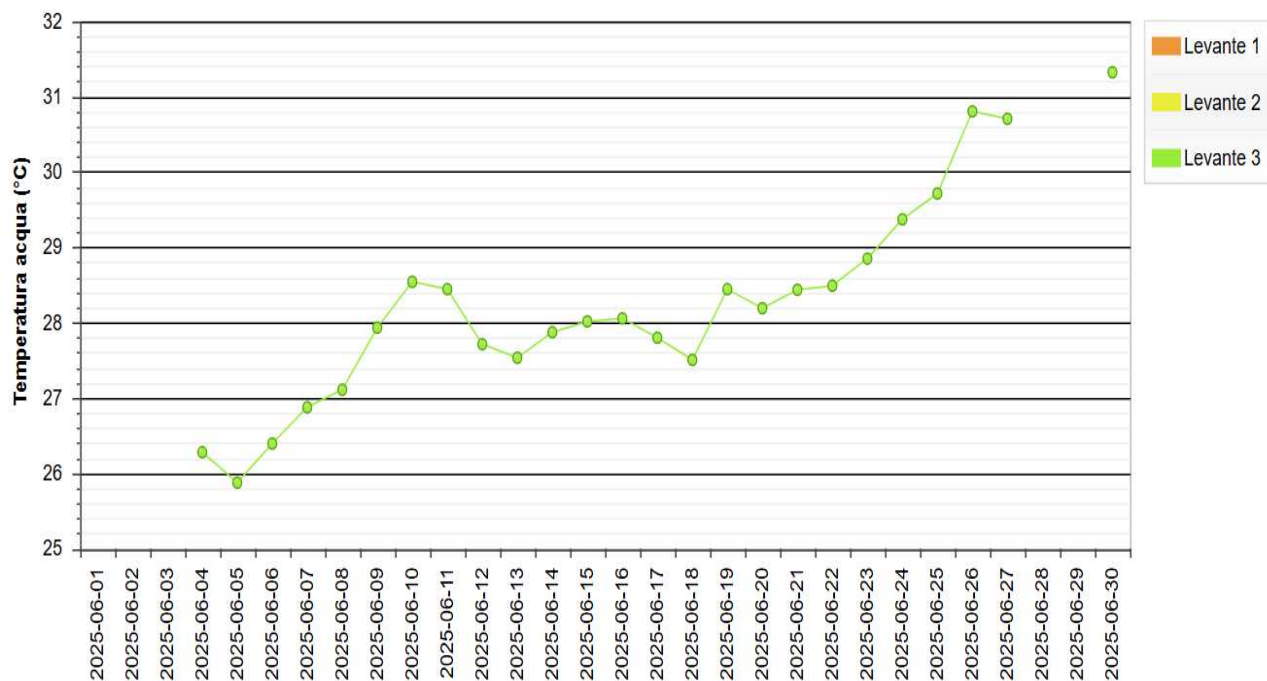
Figura 15 - Andamento medio giornaliero della Temperatura nella Laguna di Levante.
