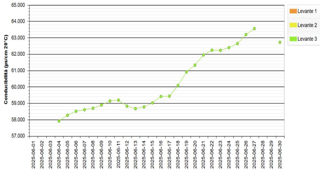
Figura 11 - Andamento medio giornaliero della Conducibilità nella Laguna di Levante.
