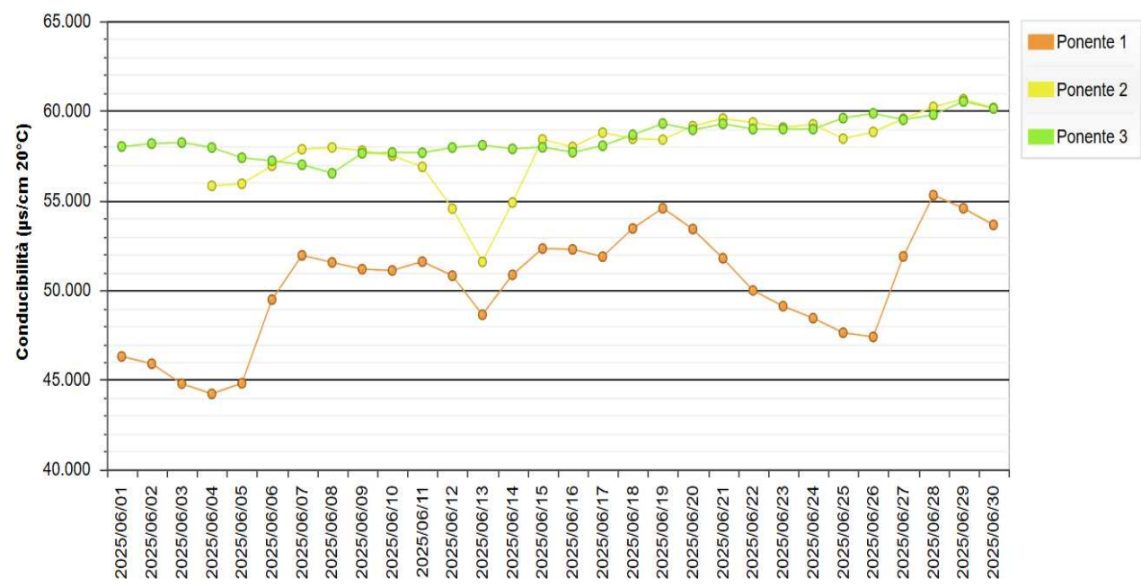
Figura 10 - Andamento medio giornaliero della Conducibilità nella Laguna di Ponente.
