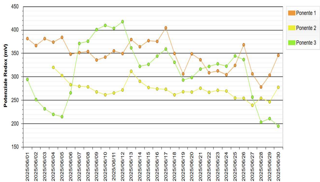
Figura 12 - Andamento medio giornaliero del Potenziale Redox nella Laguna di Ponente.
