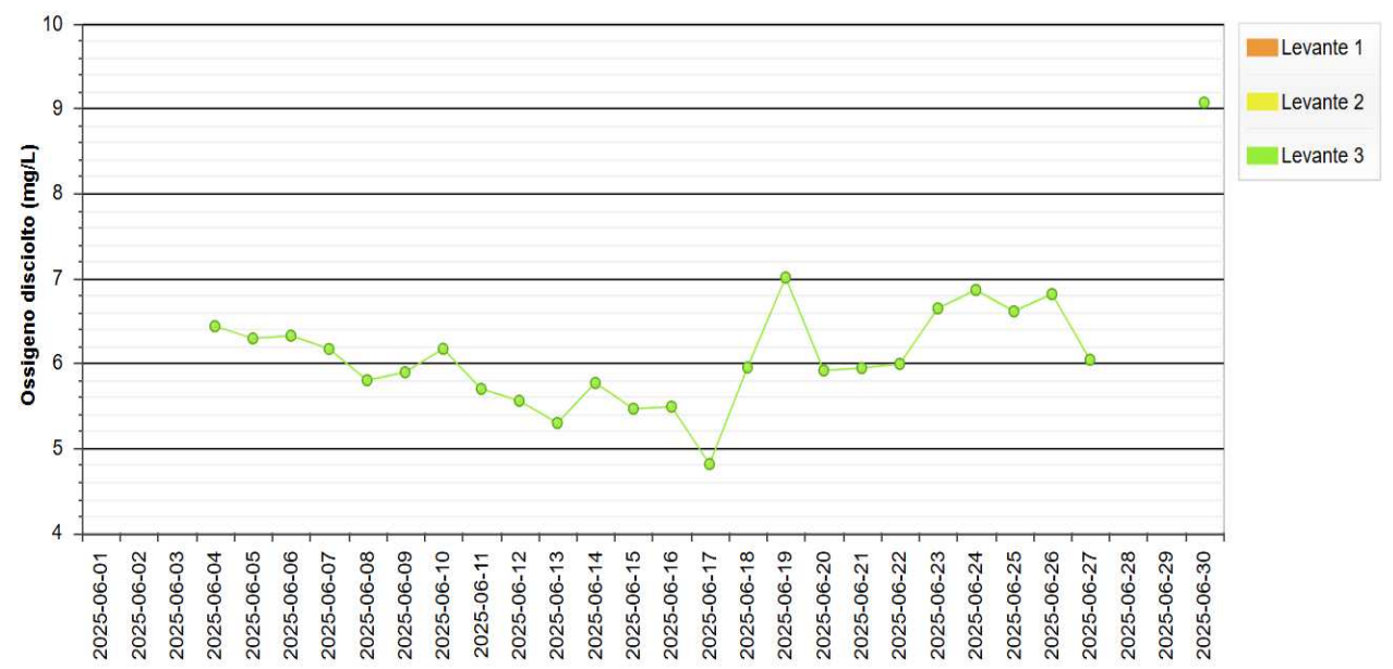
Figura 17 - Andamento medio giornaliero dell'Ossigeno disciolto nella Laguna di Levante.
