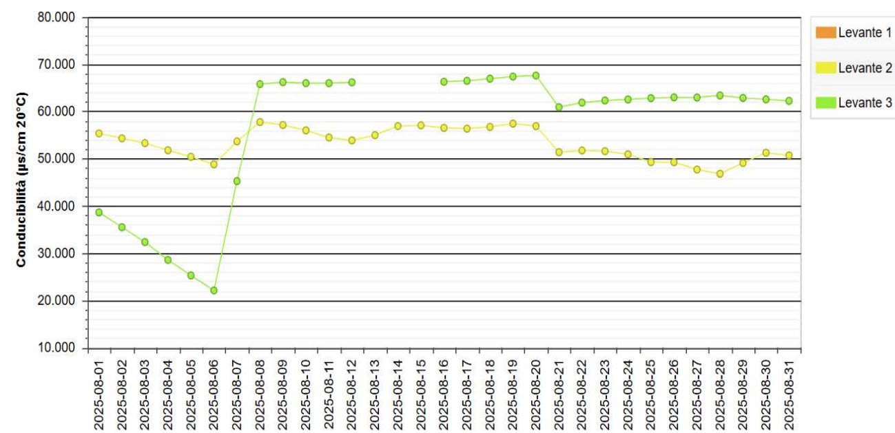
Figura 11 - Andamento medio giornaliero della Conducibilità nella Laguna di Levante.
