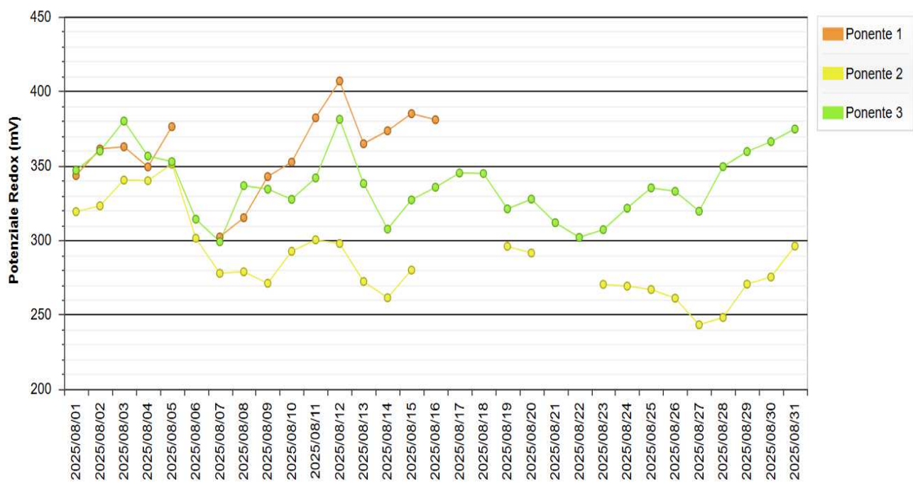
Figura 12 - Andamento medio giornaliero del Potenziale Redox nella Laguna di Ponente.
