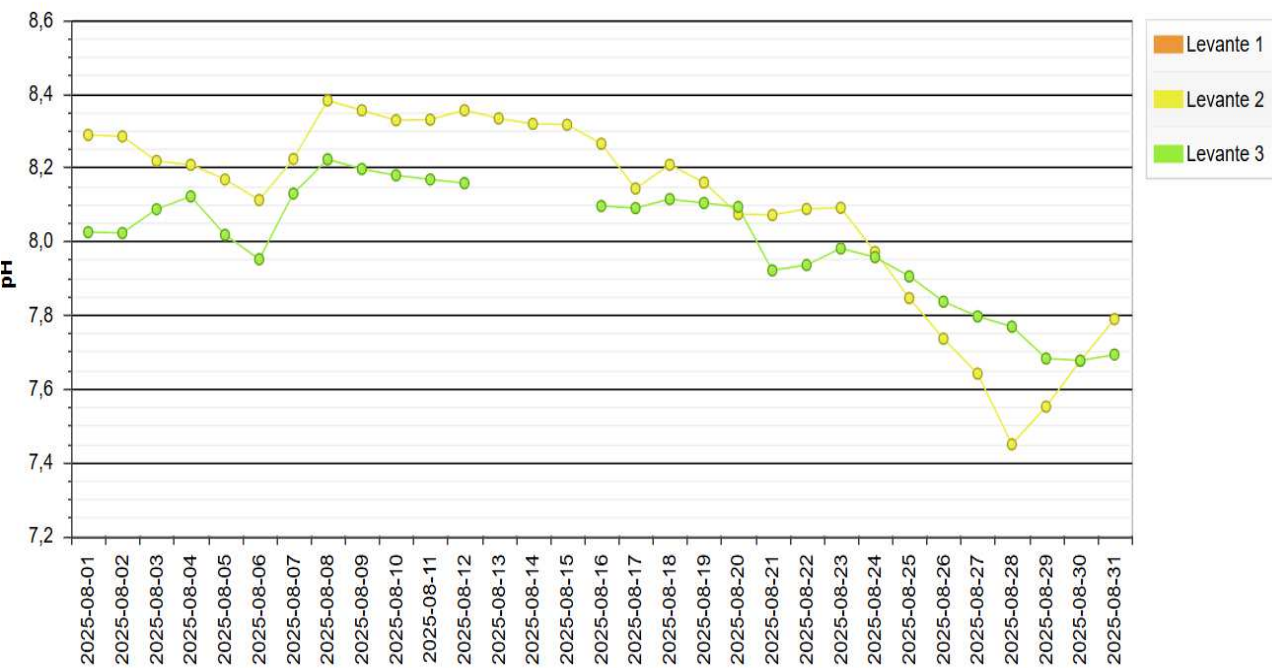
Figura 9 – Andamento medio giornaliero del pH nella Laguna di Levante.
